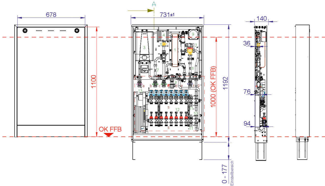
8.3 Maßzeichnung für 2 bis 8 Heizkreise im AP-Schrank
