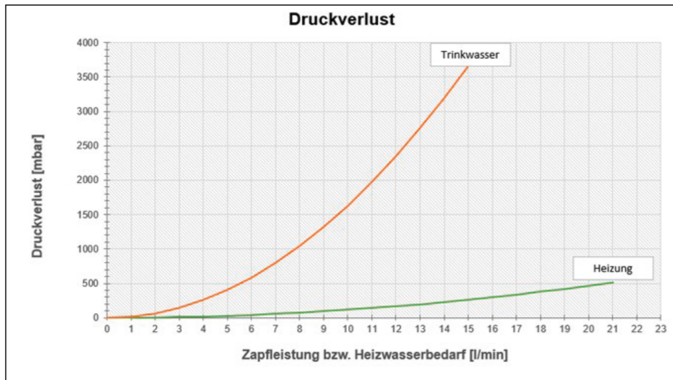
7.1 Wohnungsstation Hybrid WSHY1 Leistungsdiagramm
