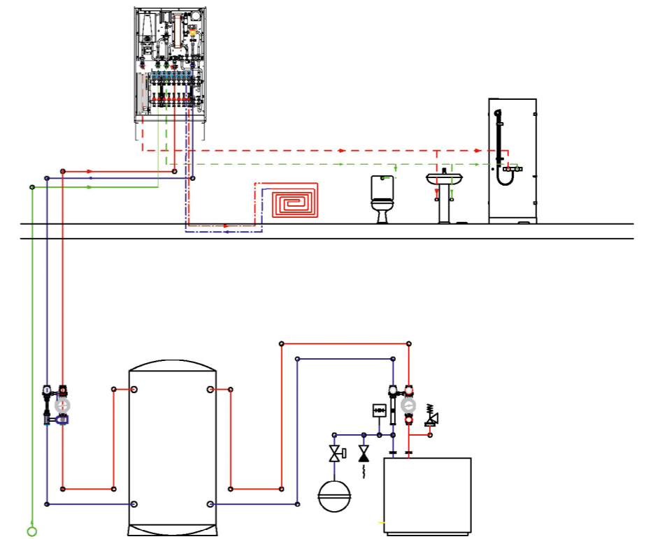
Hybrid WSHY FB-CU-UP-13,5 8 Hkr.
