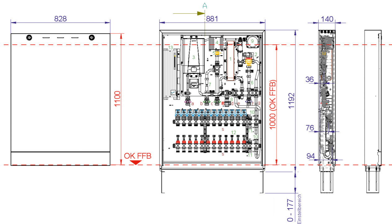
8.4 Maßzeichnung für 9 bis 12 Heizkreise im AP-Schrank
