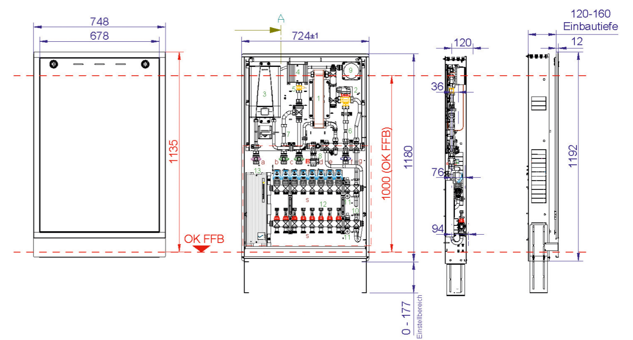
8.1 Maßzeichnung für 2 bis 8 Heizkreise im UP-Schrank
