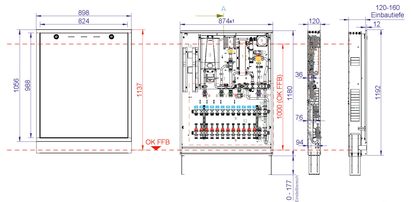
8.2 Maßzeichnung für 9 bis 12 Heizkreise im UP-Schrank
