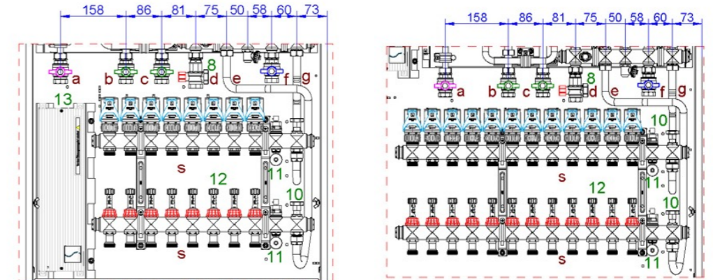
8.5 Maßzeichnung Anschlüsse und Verteiler
